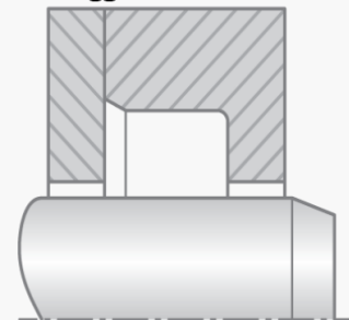
Alloggiamento chiuso
